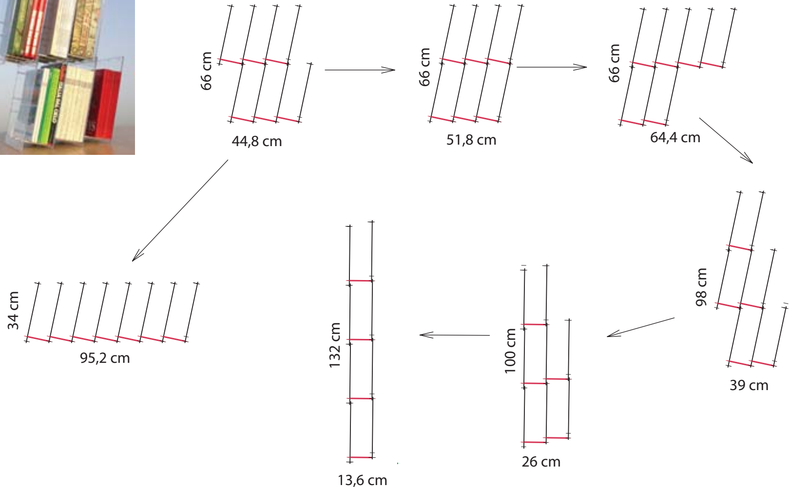
DISEGNO SCHEMATICO
